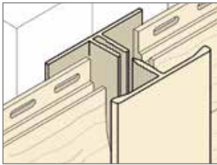
H-Profil (2-teilig)
