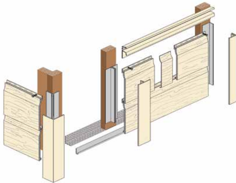
U-Profil (2-teilig)
