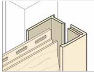
U-Profil (2-teilig)
