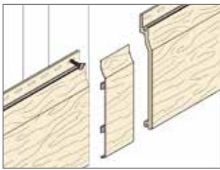
Verbinder
