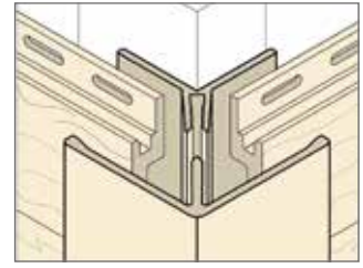
Eck-Profil (2-teilig)
