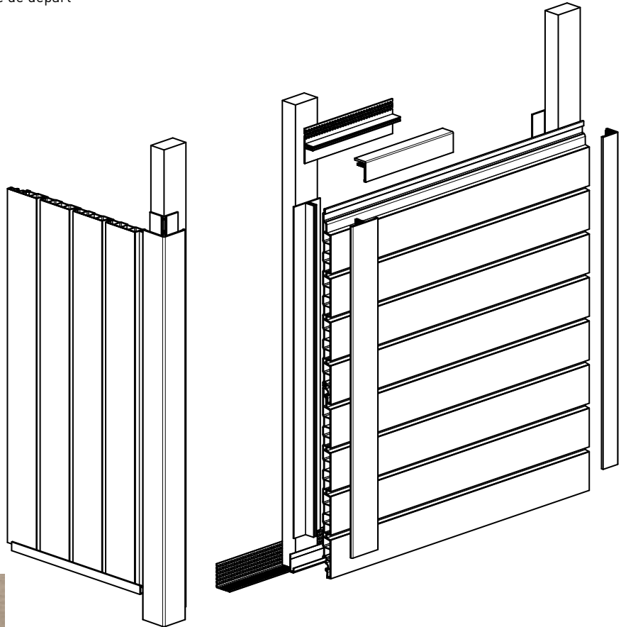
Épingle
