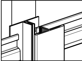
Jonction H
