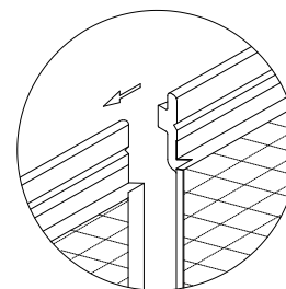
vinylit Multipaneel 2400: Seitlicher Verschluss ohne Verbinder
