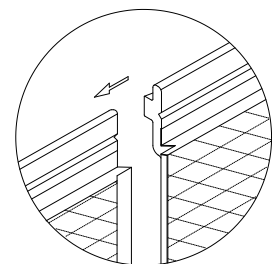
vinylit Multipaneel 2400: Seitlicher Verschluss ohne Verbinder
