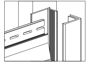
U-Profil
