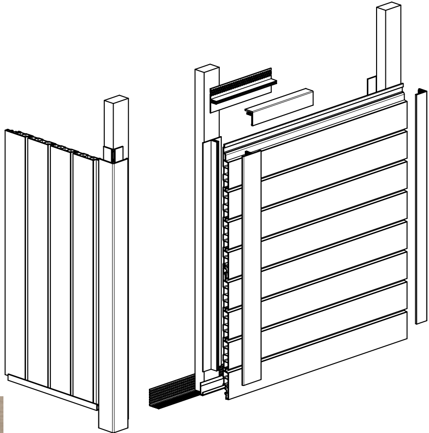
Lüftungsprofil und Starterleiste
