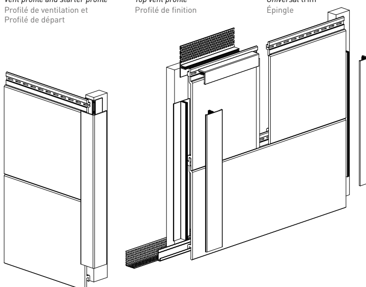
Abschlussprofil Top vent profile Profilé de finition
