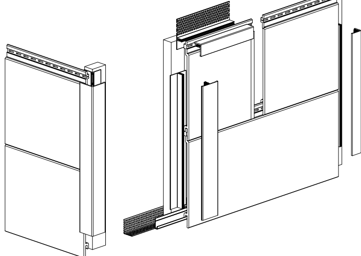
Lüftungsprofil und Starterleiste Vent profile and starter profile Profilé de ventilation et Profilé de départ
