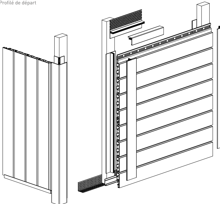
Abschlussprofil Top vent profile Profilé de finition
