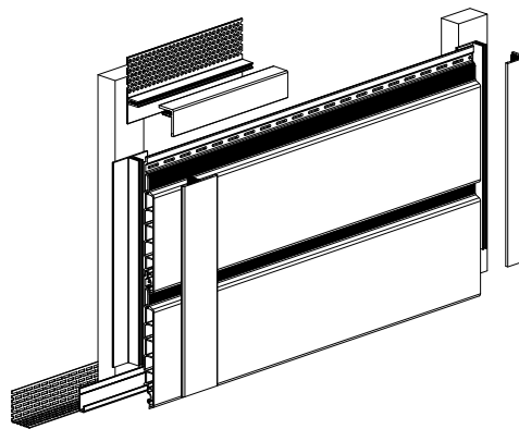
Abschlussprofil Top vent profile Profilé de finition
