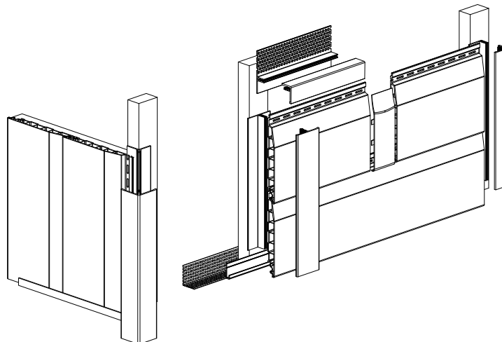
Lüftungsprofil und Starterleiste Vent profile and starter profile Profilé de ventilation et Profilé de départ
