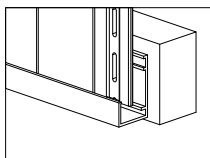
Starterleiste 6 m Starter profile 6 m Profilé de départ 6 m
