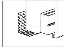
Lüftungsprofil und Distanzprofil Vent profile and space trim Profilé de ventilation et Profilé de départ
