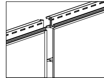
Verschluss Connection Emboîtement
