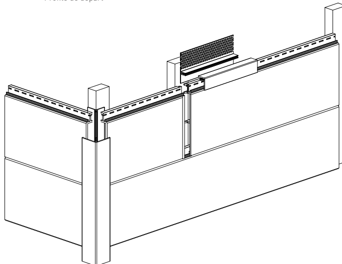
Lüftungsprofil und Distanzprofil Vent profile and space trim Profilé de ventilation et Profilé de départ
