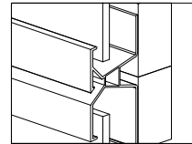
X-Profil Horizontal joint profile Profilé de jonction
