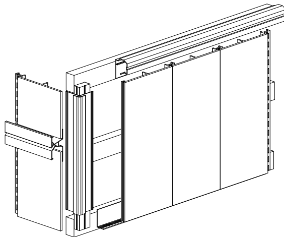
Lüftungsprofil Vent profile Profilé de ventilation
