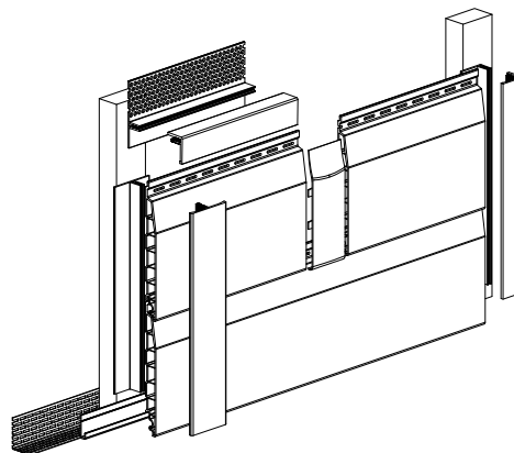
Abschlussprofil Top vent profile Profilé de finition
