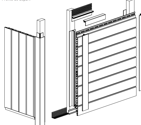
Lüftungsprofil und Starterleiste Vent profile and starter profile Profilé de ventilation et Profilé de départ
