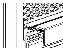
Abschlussprofil Top vent profile Profilé de finition
