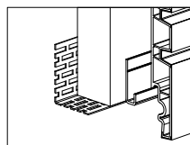
Lüftungsprofil und Starterleiste Vent profile and starter profile Profilé de ventilation et Profilé de départ
